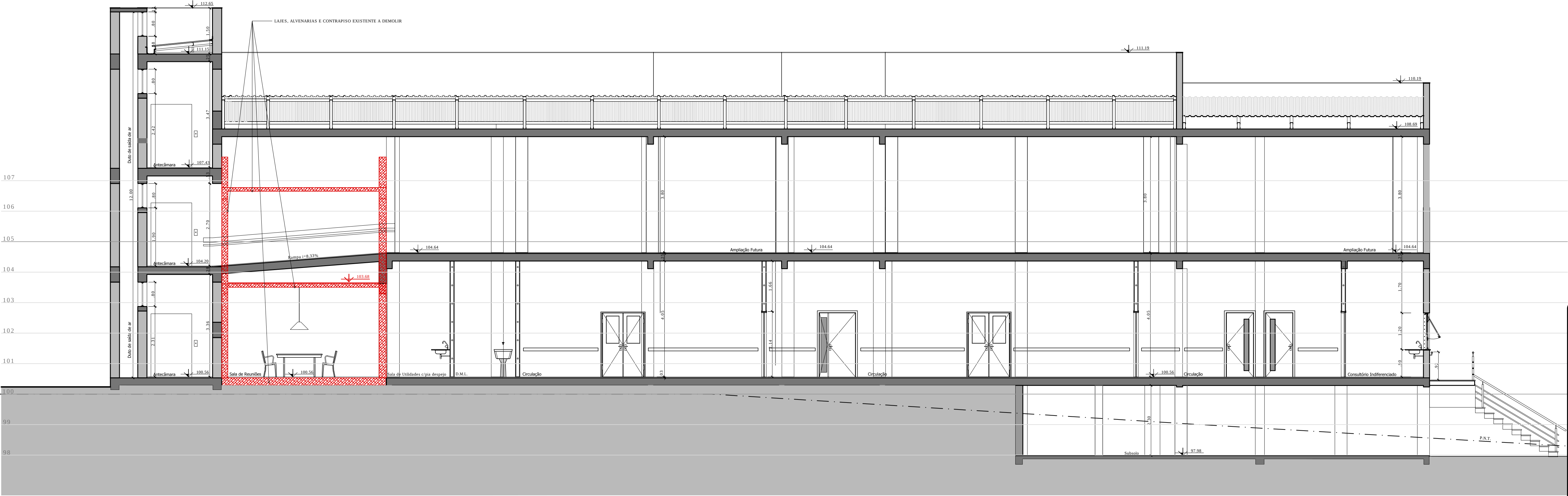
CORTE BB ESC.: 1:75
