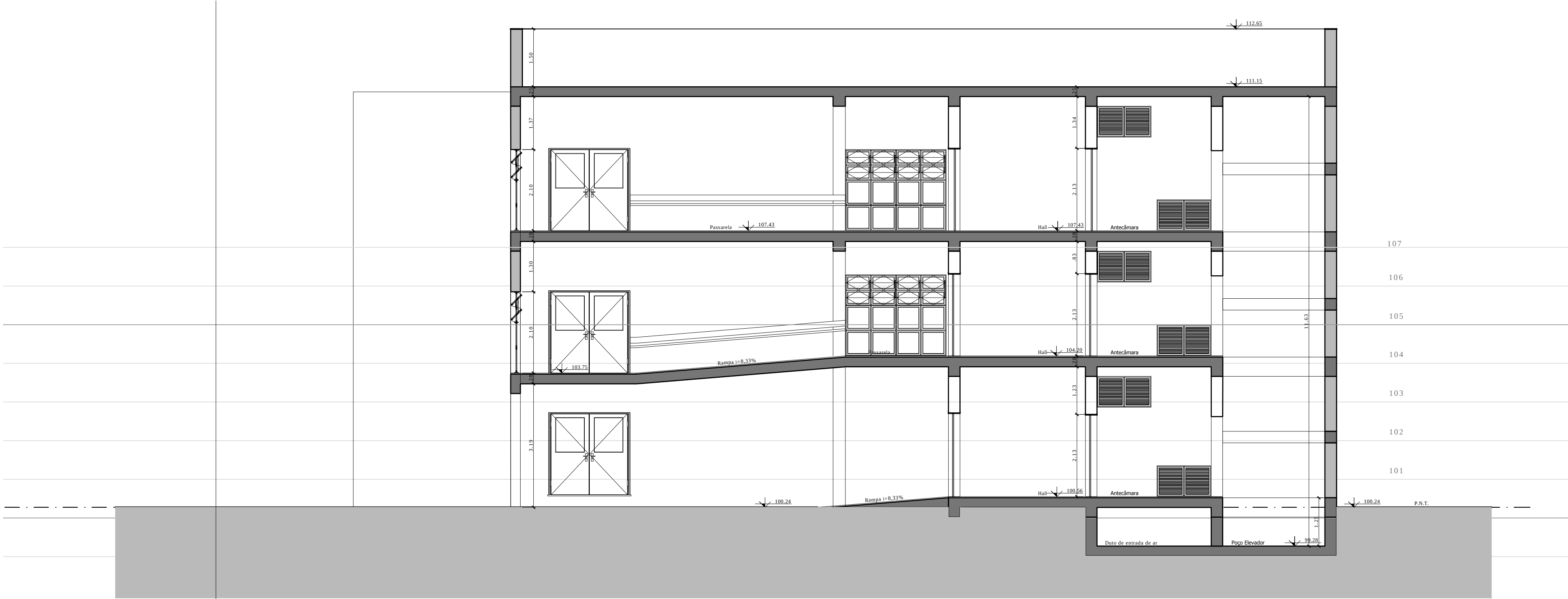
CORTE DD ESC.: 1:75
