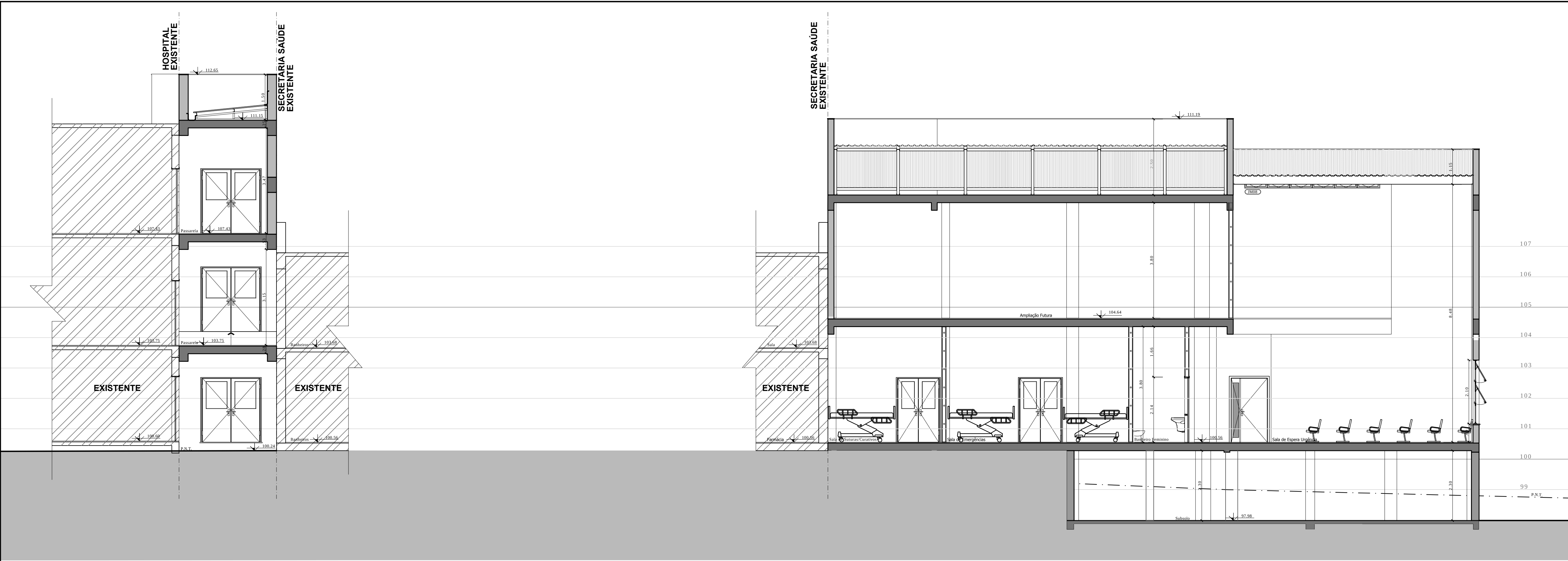
CORTE CC ESC.: 1:75
