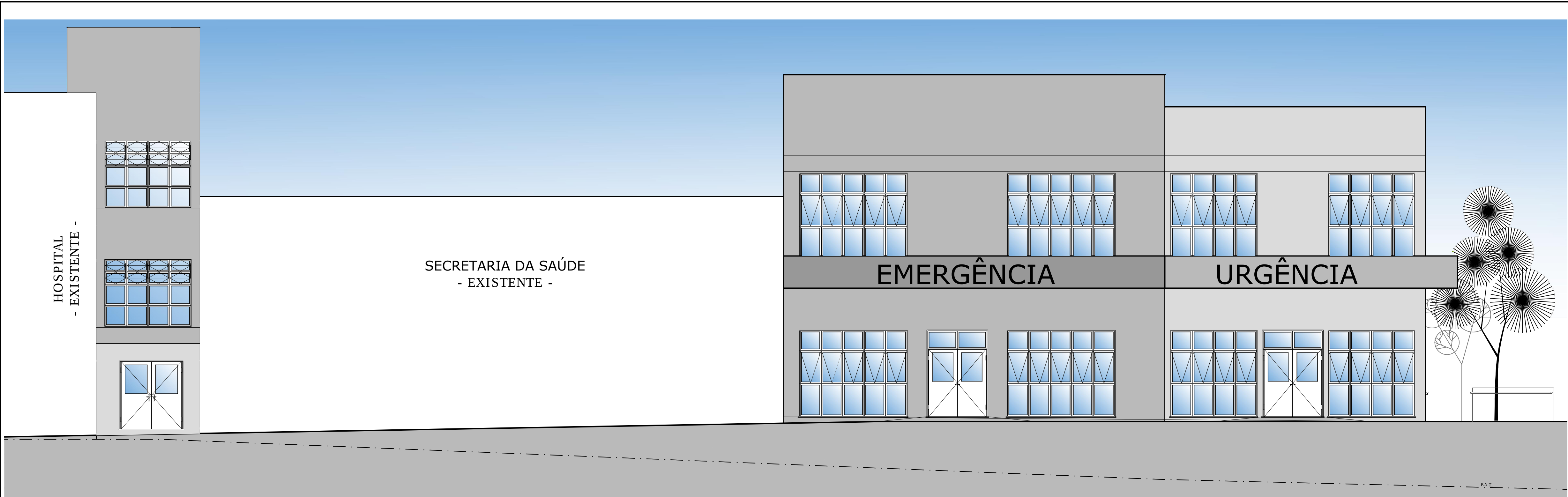
FACHADA NORTE ESC.: 1:75
