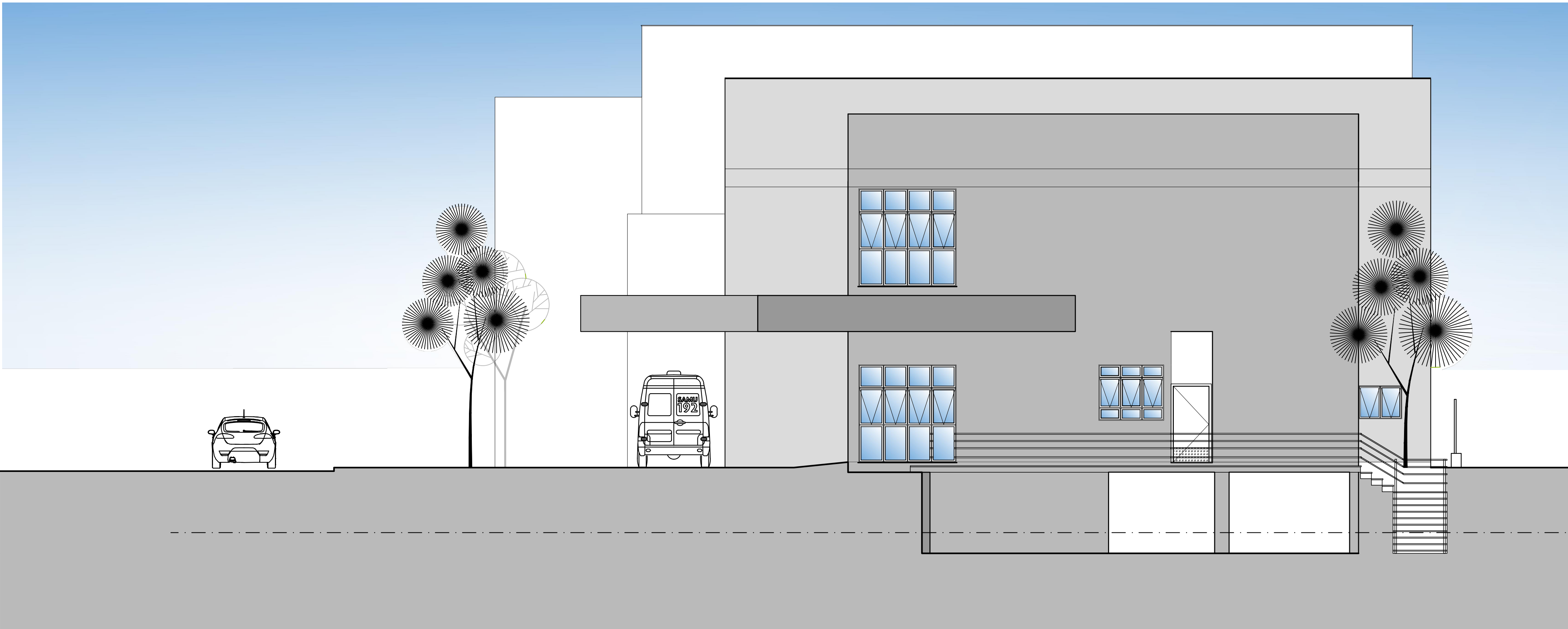
FACHADA OESTE ESC.: 1:75
